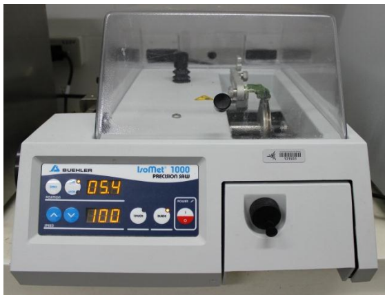
Figura 5. Aparelho de precisão Isomet 1000 Precision Saw (Bulher Ltda, Lake Bluff, IL, USA).
