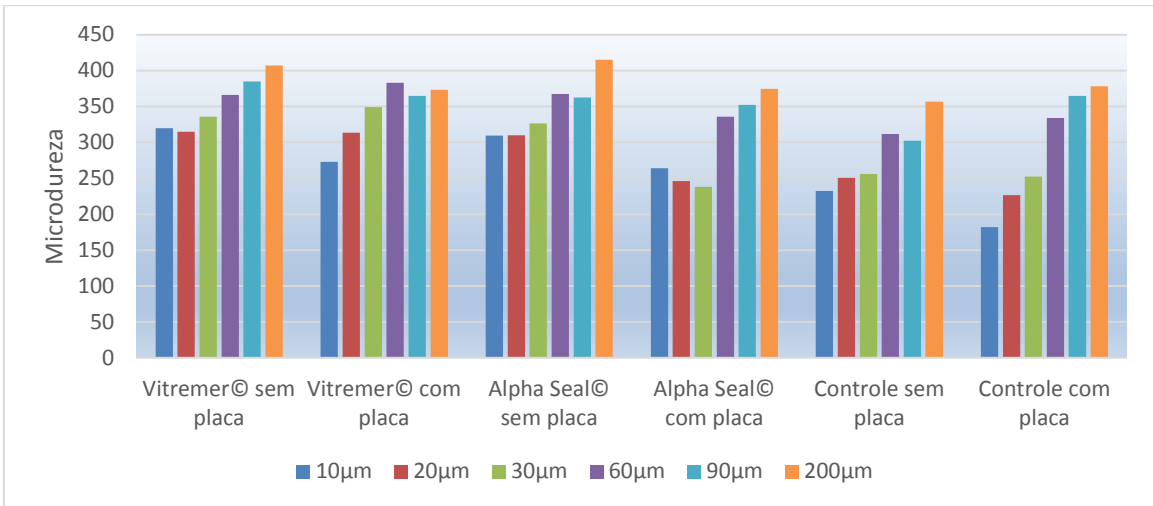
Figura 13. Desempenho dos grupos experimentais, medidas por microdureza longitudinal, considerando a fileira 100µm.
